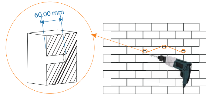
Taladro Ø10 mm b) (Profundidad: 60 mm)
